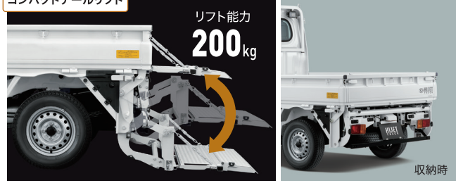
スイングアーム式テールゲート
