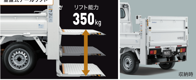
垂直式テールゲート
