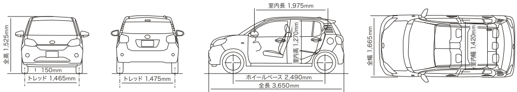
ブーン寸法図 車種: X "L"パッケージ(2WD)
